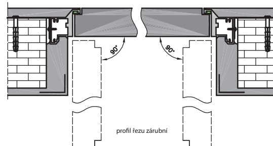
DVEŘE S POLODRÁŽKOU OTEVÍRAVÉ DOVNITŘ
