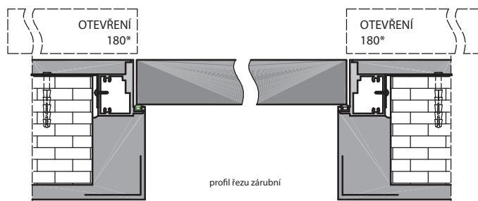
BEZPOLODRÁŽKOVÉ KŘÍDLO OTEVÍRAVÉ VEN
