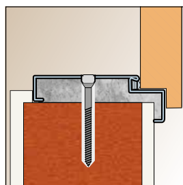
MONTÁŽ NA HMOŽDINKY
