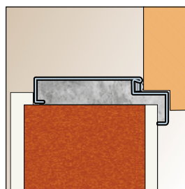
MONTÁŽ BEZ DODATOČNÝCH KOTVÍCÍCH PRVKOV
