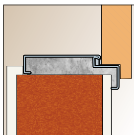
MONTÁŽ BEZ DODATEČNÝCH KOTVÍCÍCH ELEMENT
