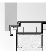
montáž na sádkartonové stěně
