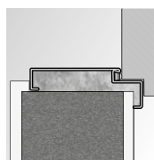
AGAT Montáž bez dodatečných kotvicích elementů.
