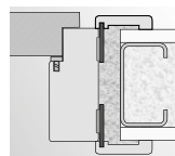
montáž do pěny do zděné stěny
