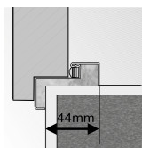
rohová zárubně malá
