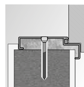
OPAL Montáž s pomocí kotev
