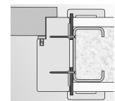
montáž na vruty do stěny ze sádkokartonové desky
