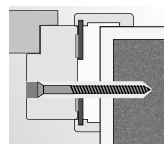
montáž do pěny a kotvy do zděné stěny
