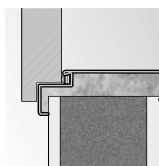
montáž bez dodatečných kotvicích prvků
